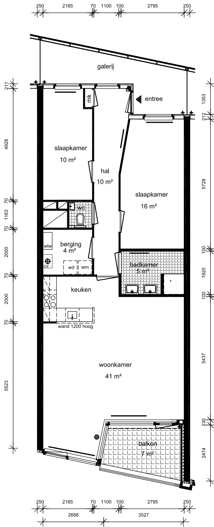
PLATTEGROND
