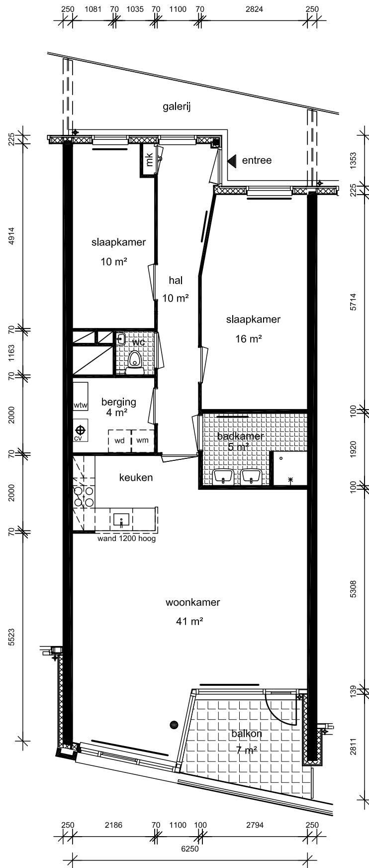
PLATTEGROND
