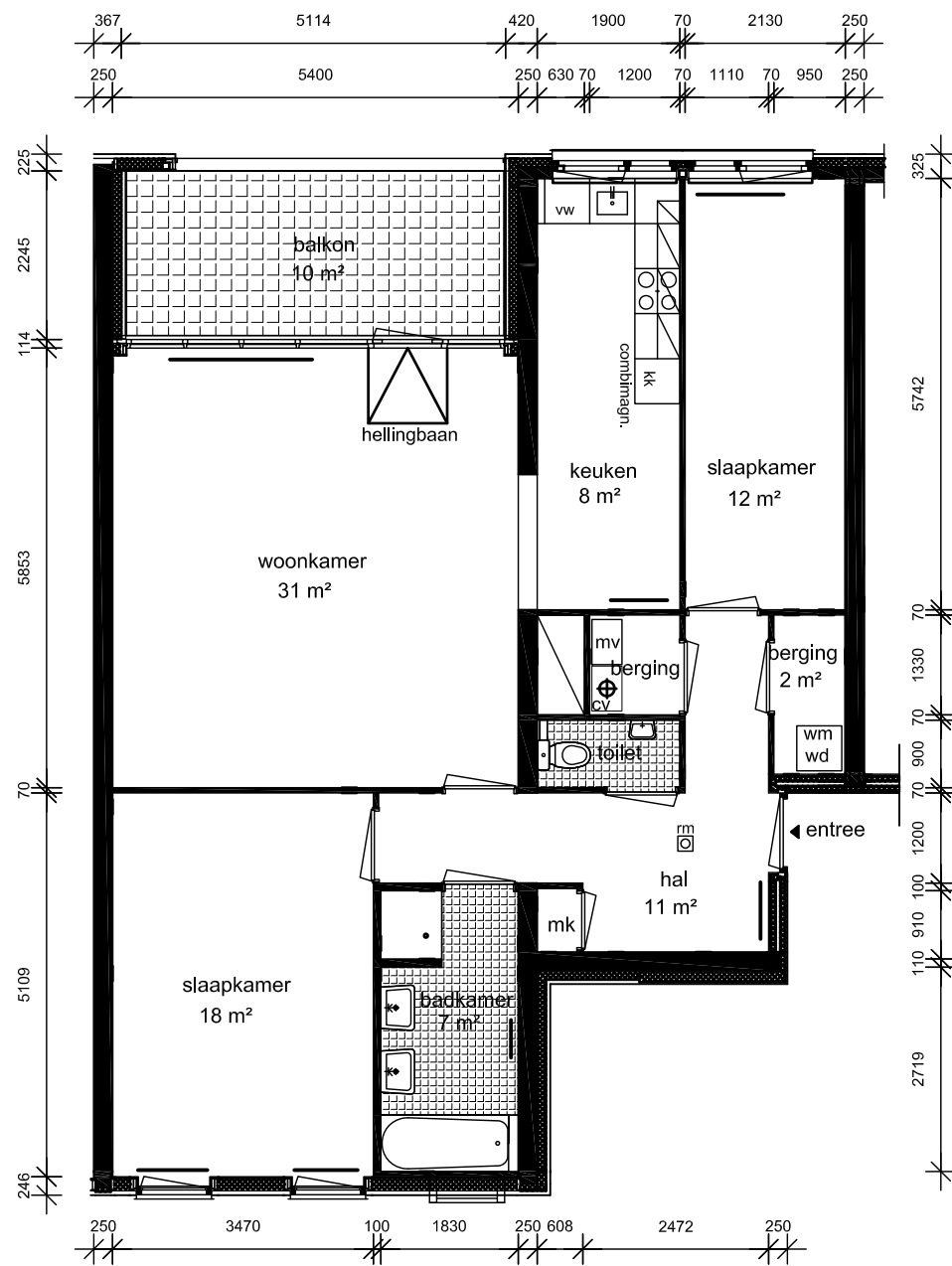
PLATTEGROND
