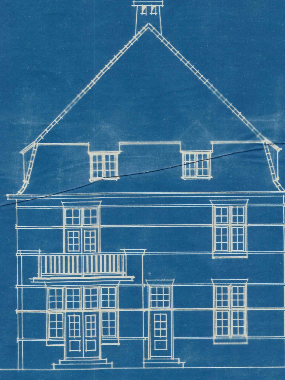
ACHTER-GEVEL
