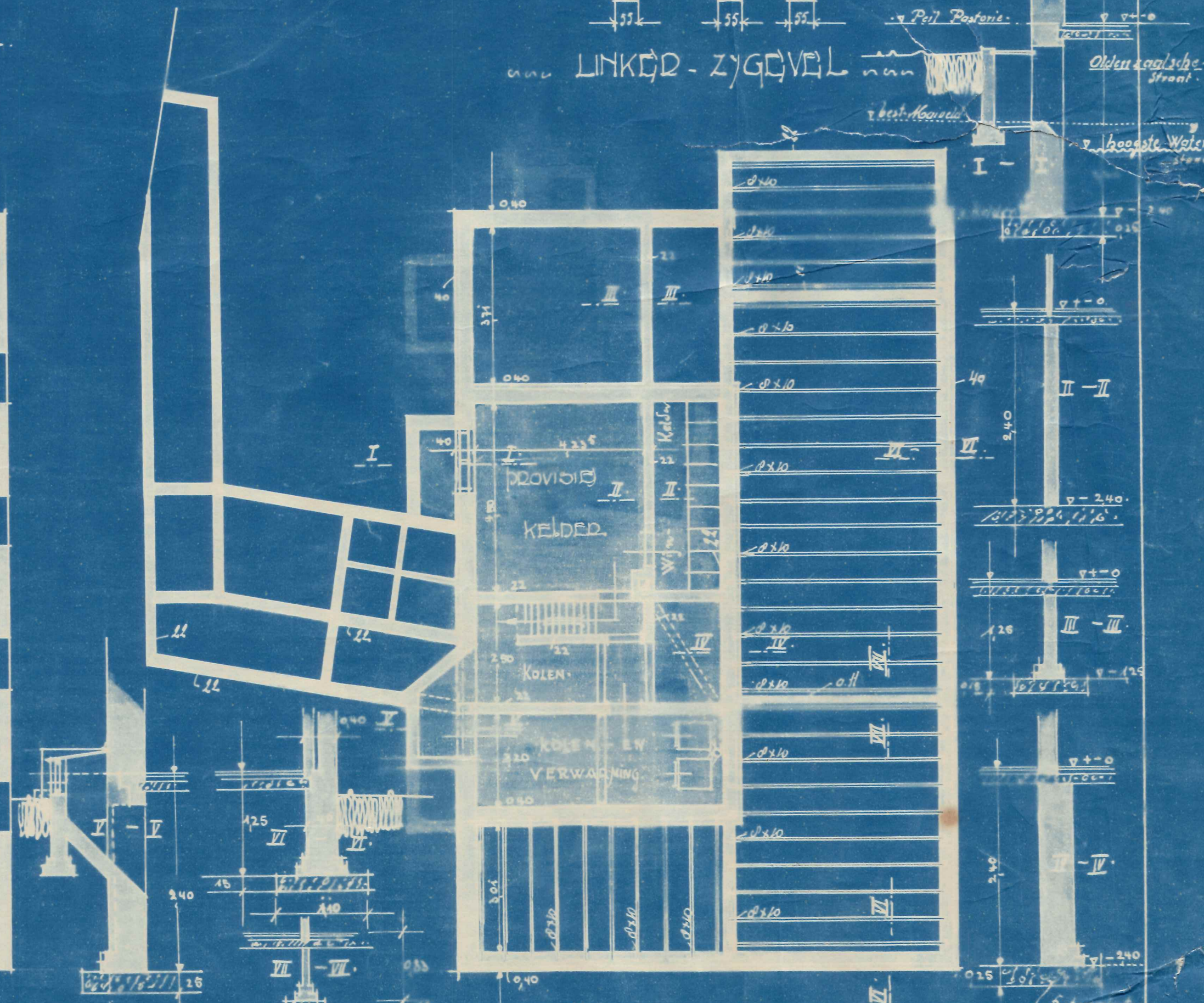
Kelder-plan
