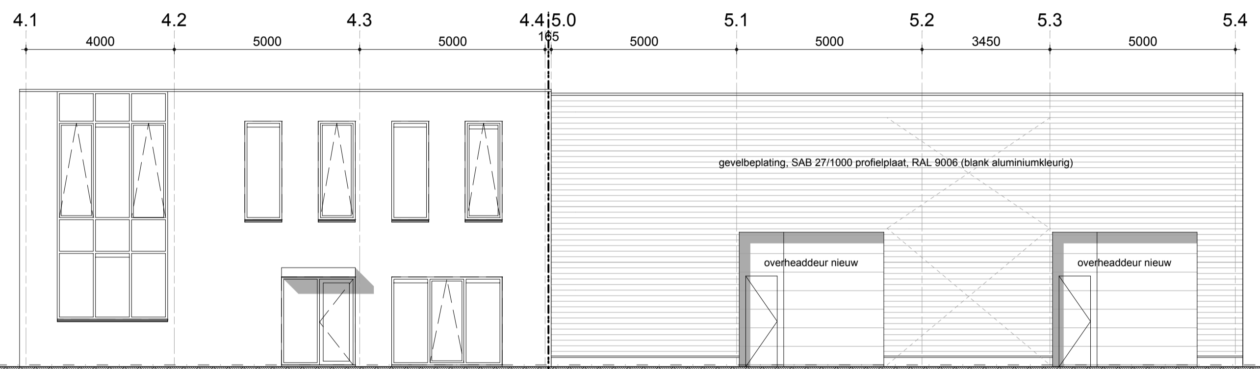
kavel 4 - ongewijzigd VOORGEVEL
