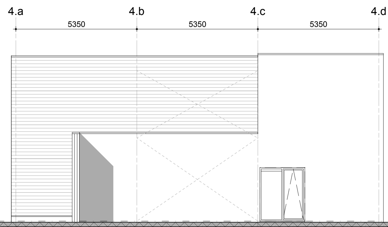
kavel 4 - ongewijzigd LINKER ZIJGEVEL
